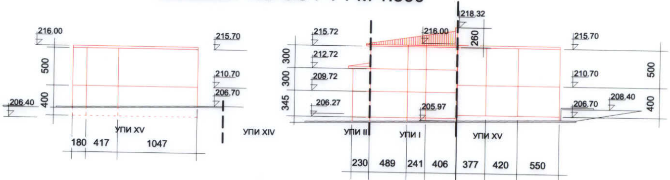
СИЛИУЕТ ПО ОС А-А1 М 1:500
