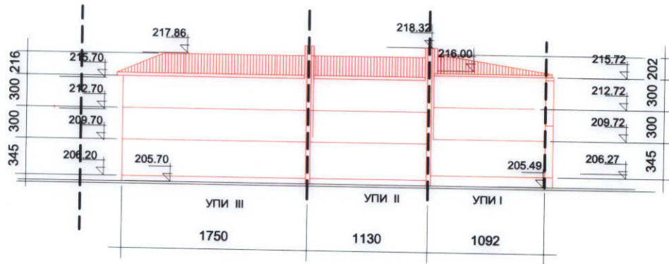
СИЛИУЕТ ПО ОС Г-Г1 М 1:500
