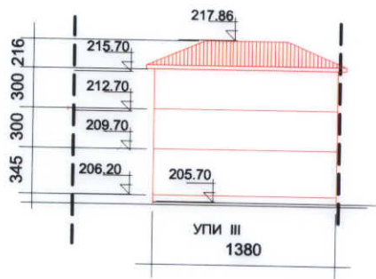
СИЛИУЕТ ПО ОС Д-Д1 М 1:500
